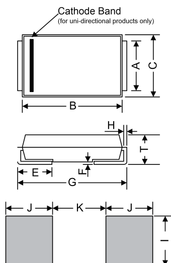
DO-214AB (SMC)
