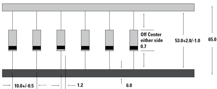
Tape (Unit:mm)
