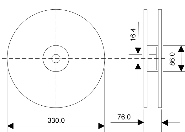
Reel (Unit:mm)
